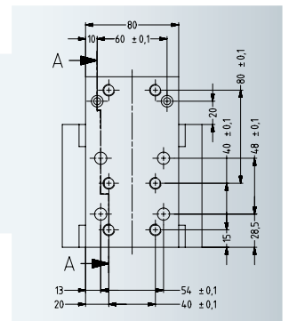
ER-108194 RCS5 Greifer mit Lasthaken
