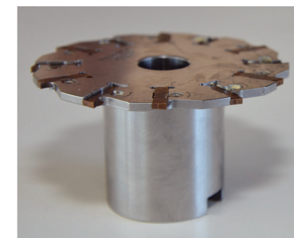
3 Die Wendeschneidplatten des kompakten, vielzahnigen Standardfräasers GN18 zum Schlitz- und Trennen sind formschlüssig gegen den Uhrzeigersinn fixiert. Deshalb ist er besonders sicher © Hanser
