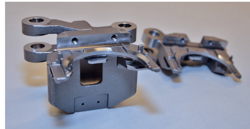
2 In jedes der jährlich gut 5000 Kettenglieder im neuen Design (links) ist eine Nut einzubringen (unter dem Halbrund). Rechts ein übliches Teil, das zwar kleiner ist, dem aber der zusätzliche Schutz vor Verunreinigungen fehlt © Hanser
